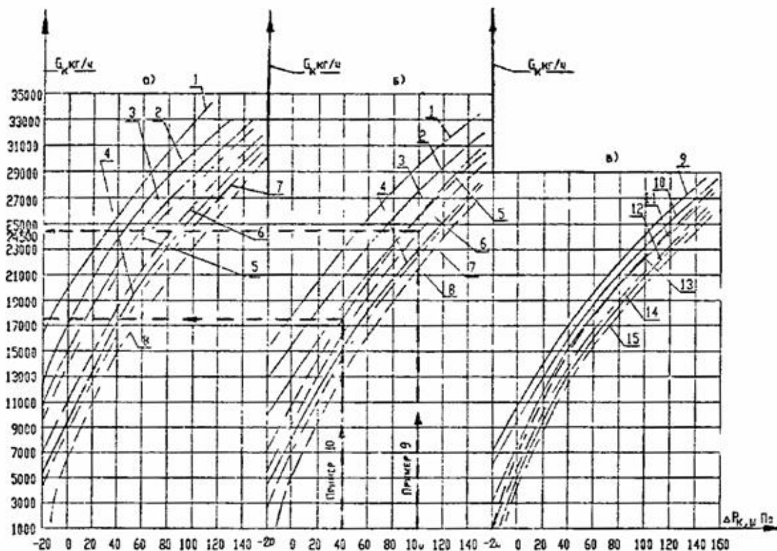
Рис. 11 а, б, в. Планировка Б. Расход воздуха G_k , кг/ч для незадымляемой лестничной клетки 2-го типа в зависимости от разности давлений между лестничной клеткой и лифтовой шахтой \Delta P_{k,л} на верхнем этаже и от давления в лифтовой шахте на 1-ом этаже, P_{ш1} , Па
