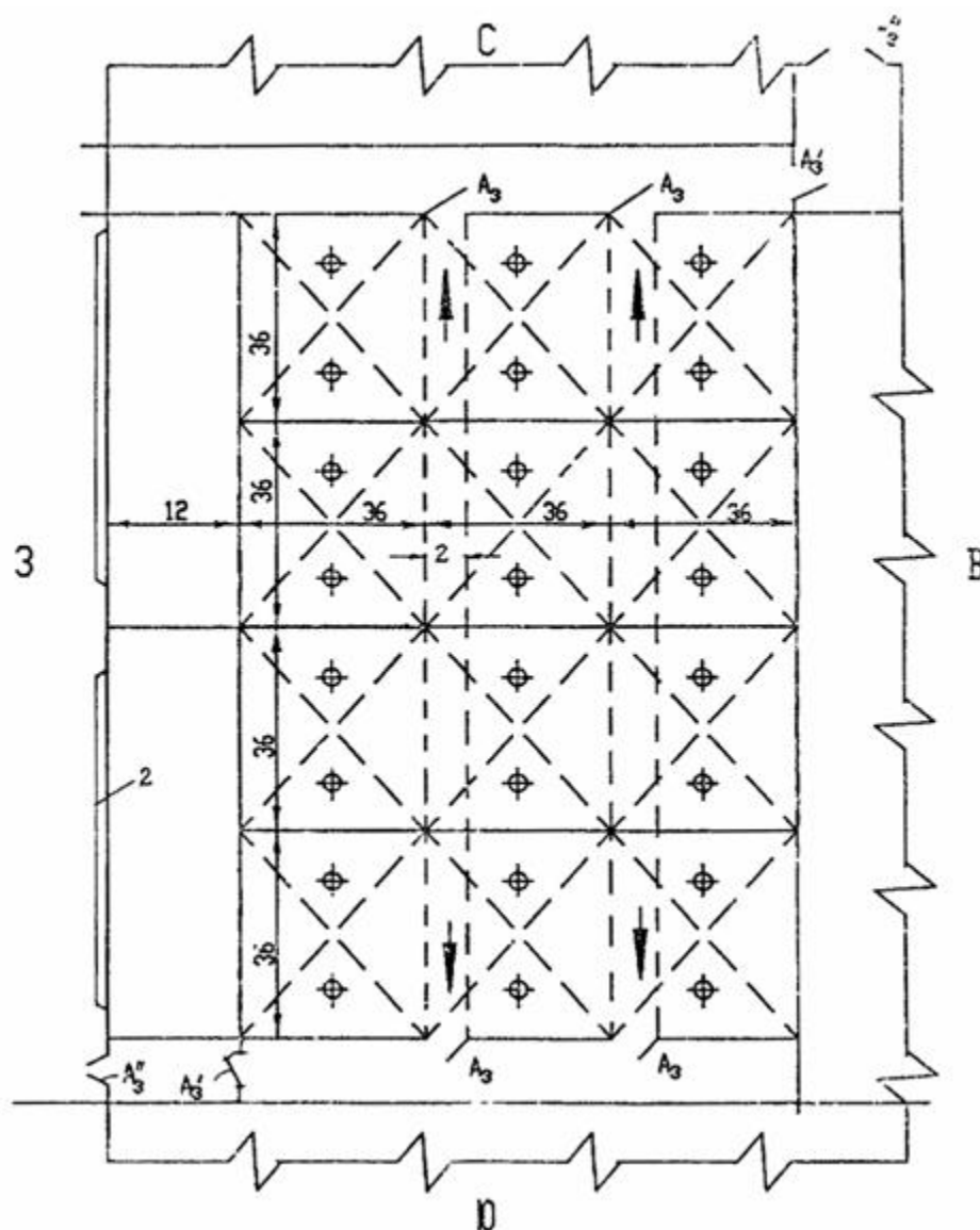
Рис. 8 - к примеру 5. План помещения с размещением шахт, фрамуг и дверей эвакуационных выходов:
