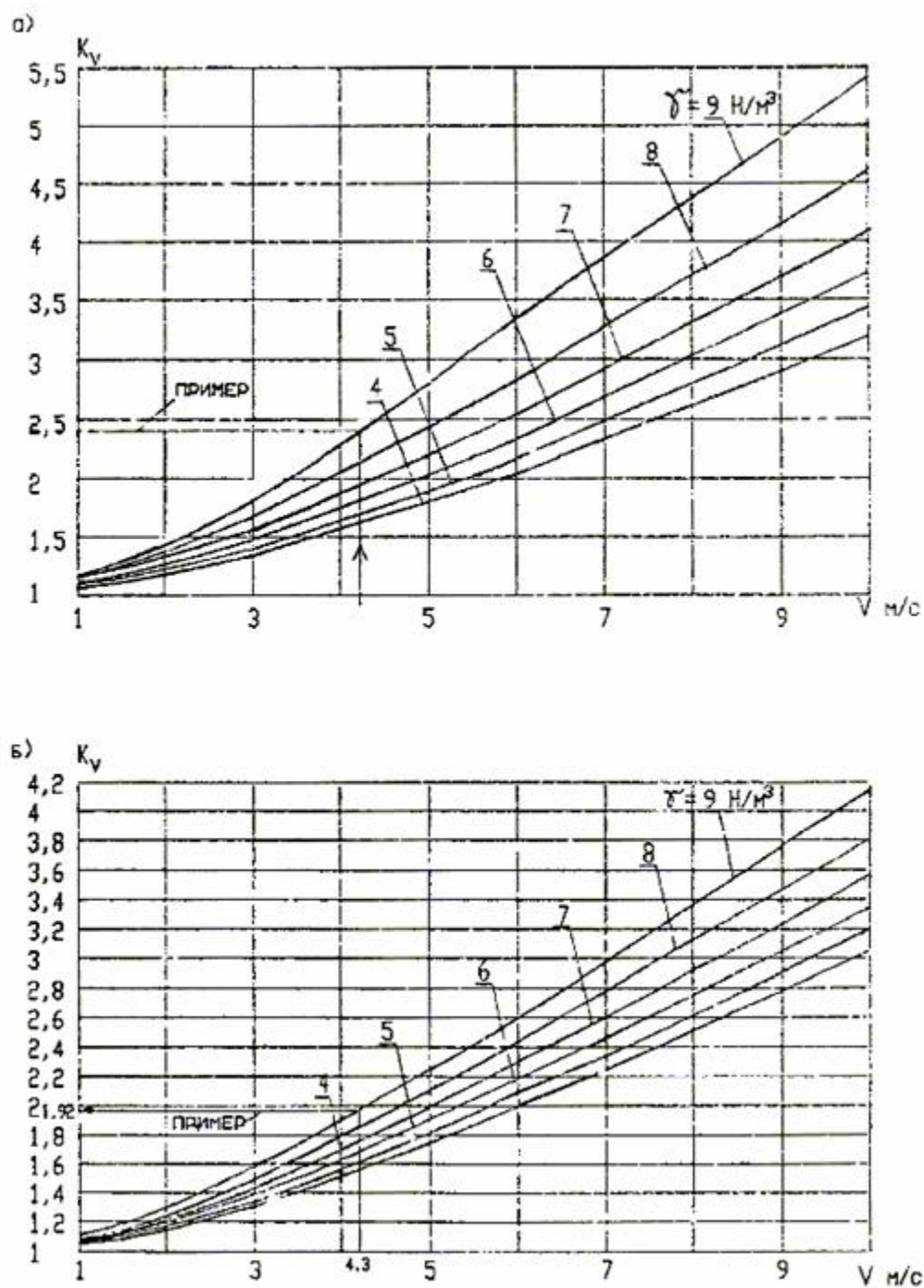
Рис. 15. Планировка Г. Расход наружного воздуха, G_K , кг/ч, в незадымляемую клетку 2-го типа при планировке Г в отделенную «рассечкой» нижнюю зону
