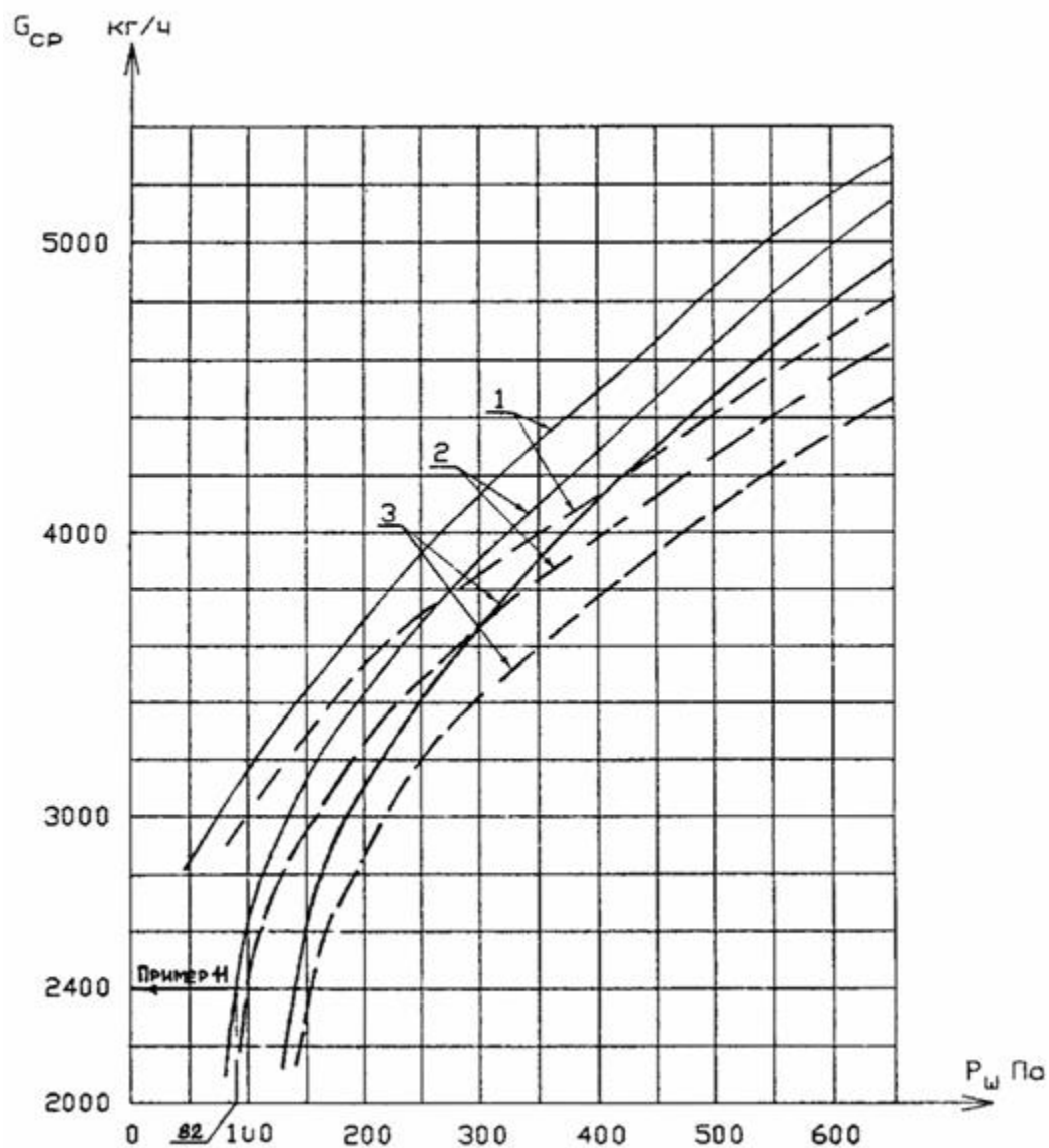
Рис. 14. Планировка Г. Средний расход наружного воздуха G_{cp} , кг/ч, на каждый этаж со 2-го по верхний в зависимости от давления в шахте на верхнем этаже 11 -
