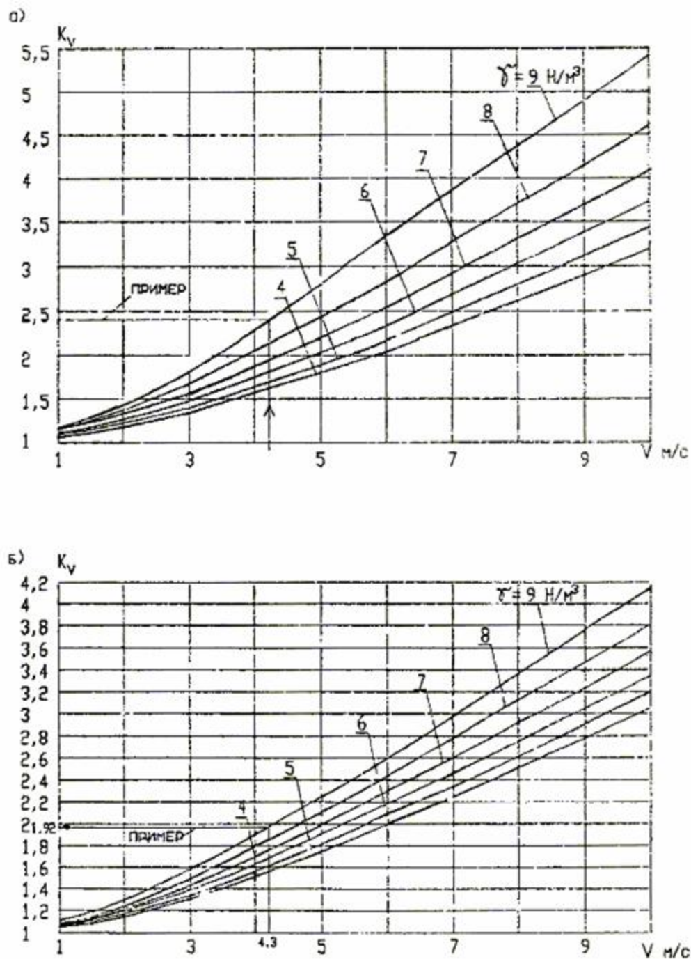
Рис. 4. График для определения коэффициента K_V в зависимости от скорости ветра, V м/с, и удельного веса дыма H/m^3 :
