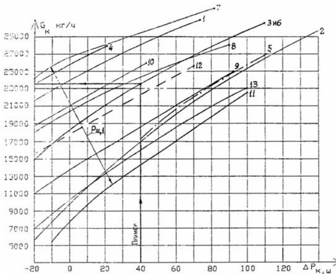
Рис. 13. Планировка В. Расход воздуха, G_k , кг/ч, в лестничную клетку 2-го типа в зависимости от разности давлений \Delta P_{k,ш} на уровне верхнего этажа и давления в лифтовой шахте на 1-ом этаже P_{ш,1} , Па
