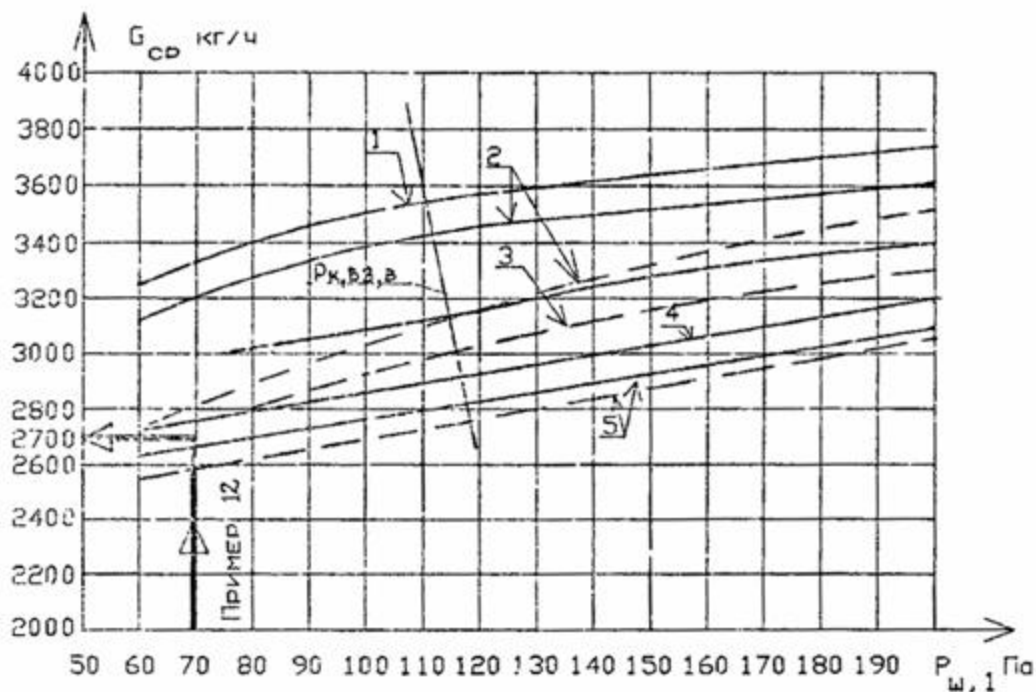
Рис. 17. Планировка В. Средний расход наружного воздуха, кг/ч, для верхней зоны здания из 5-ти \frac{3}{4} или 13-ти --- этажей, с внутренним переходом в нижнюю зону, в зависимости от давления воздуха в лифтовой шахте на 1-ом этаже P_{ш,1} Па и давлении в верхней зоне на верхнем этаже P_{к,вз,б} Па равно для кривой 1-220 Па, кривой 2-180, кривой 3- 50, 4-90 и 5-60 Па
