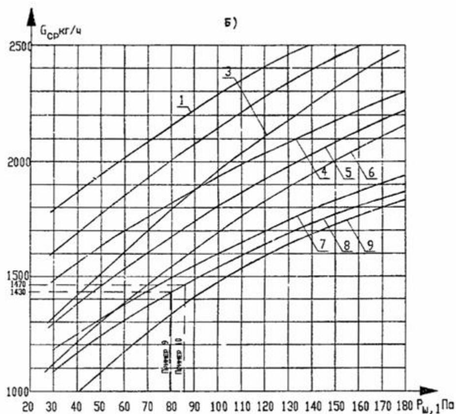
Рис. 106. Средний расход воздуха, G_{ср} кг/ч, на каждый этаж со 2-го по верхний в зависимости от давления воздуха в лифтовой шахте на 1-ом этаже, P_{ш1} Па, числа дверей на этаже и температуры наружного воздуха в холодный период года параметры Б для 15-20 этажного здания
