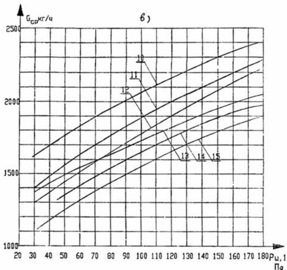
Рис. 10в. Средний расход воздуха, G_{cp} кг/ч, на каждый этаж со 2-го по верхний в зависимости от давления воздуха в лифтовой шахте на 1-ом этаже, P_{w1} Па, числа дверей на этаже и температуры наружного воздуха в холодный период года параметры Б для 21-27 этажного здания
