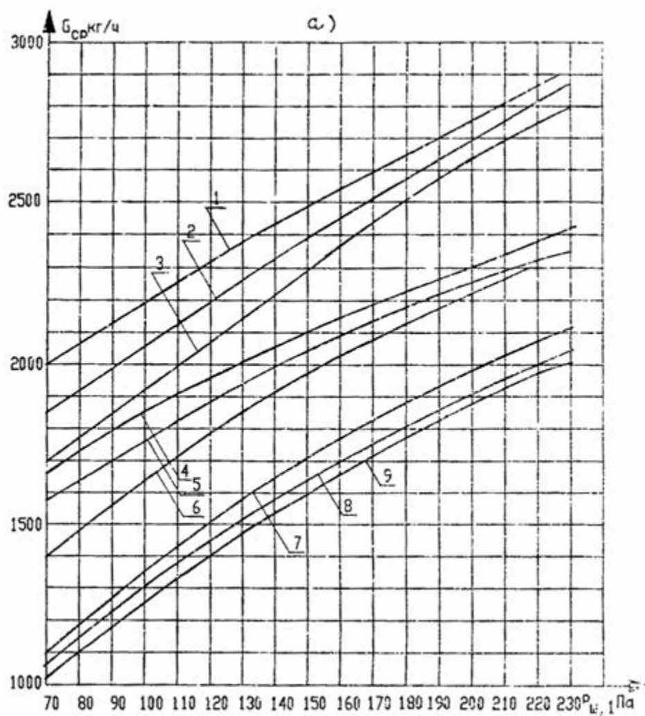
Рис. 10а. Средний расход воздуха, G_{cp} кг/ч, на каждый этаж со 2-го по верхний в зависимости от давления воздуха в лифтовой шахте на 1-ом этаже, P_{w1} Па, числа дверей на этаже и температуры наружного воздуха в холодный период года параметры Б для 10-14этажного здания
